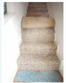
直部は下から上へグリッパーに 引っかけながらつなげて張る
